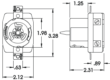
Receptacle
